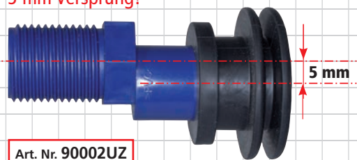
Urinal Zulauf-Garnitur für UP 1/2" mit Dichtung 5 mm Versprung!
