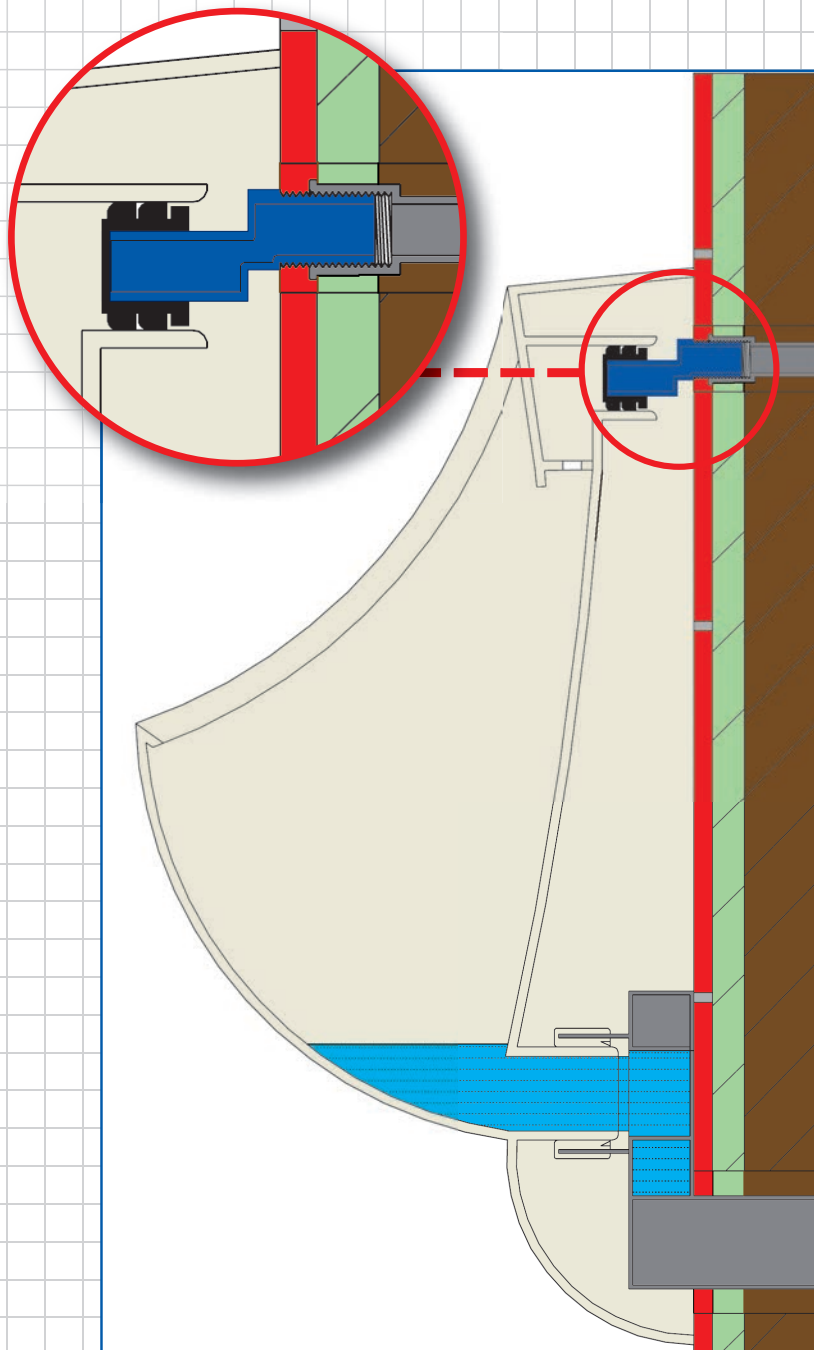
Urinal Zulauf-Garnitur für UP 1/2" mit Dichtung 5 mm Versprung!
