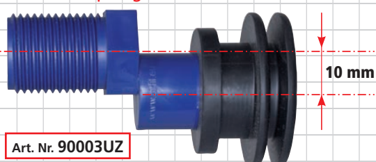
Urinal Zulauf-Garnitur für UP 1/2" mit Dichtung 10 mm Versprung!
